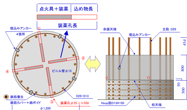
図-2 杭頭部模擬試験体: 試験体1
