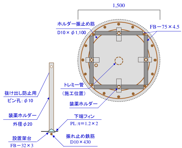
図-1 装薬ホルダー: 水平フィン付(前施工・豎管方式)
