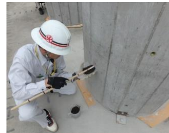
写真-5 タンピング (試験体1)
