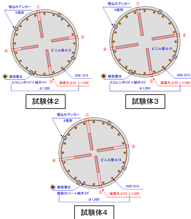
図-3 杭頭部模擬試験体：試験体2～4
