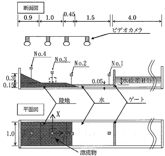
図-1 漂流実験の模式図
