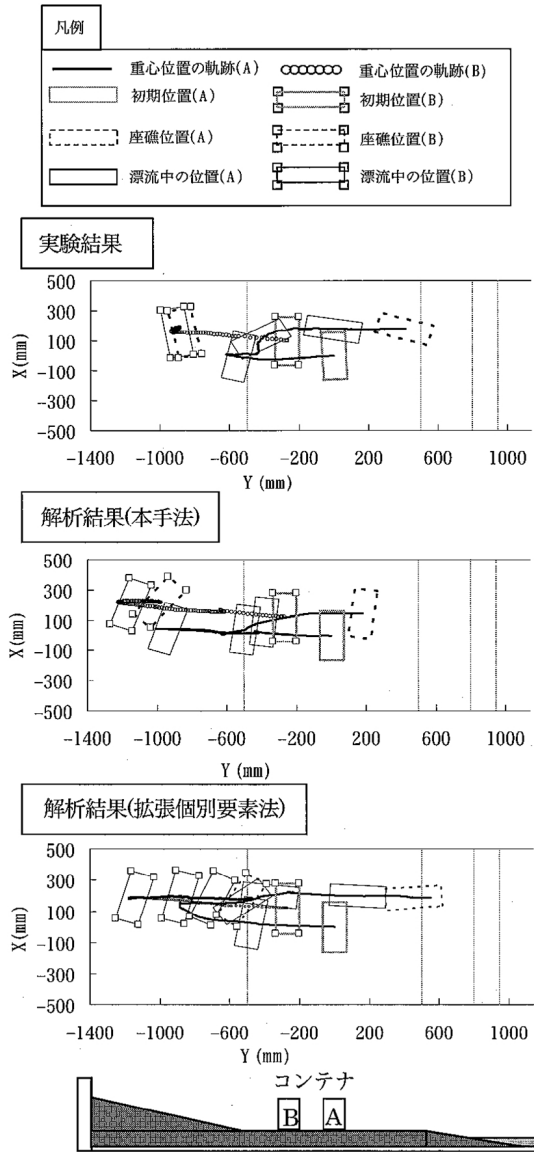
図-4 漂流軌跡の比較(コンテナ2基同時配置, 並列)
