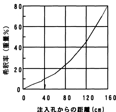
図-12 注入センターからの距離と薬液の希釈率の関係
