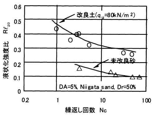
図-7 改良土の繰返し載荷試験結果例
