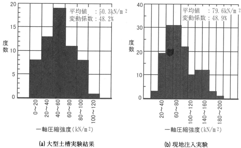
図-1.3 大型土槽実験と現場注入実験における q_u のヒストグラムの比較
