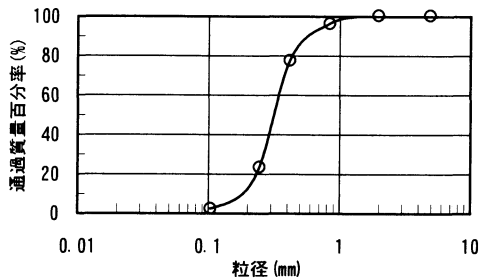
図-5 新潟砂の粒度分布
