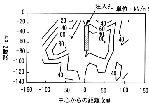
図-9 土槽内の q_u の分布(28日後)
