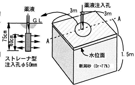
図-8 大型土槽注入装置
