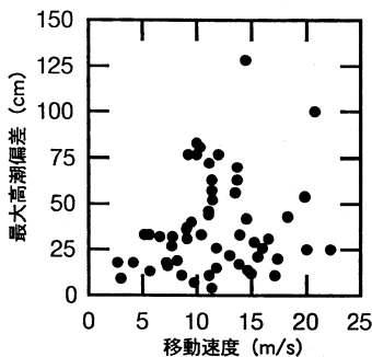
図-3 移動速度と高潮偏差の関係
