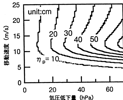
図-9 \eta_p の分布
