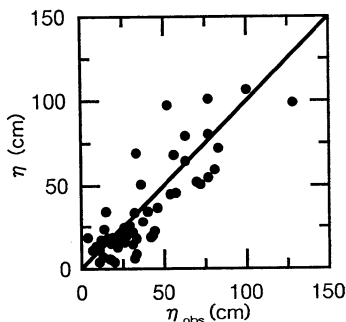
図-7 推定式による高潮偏差と観測値の比較
