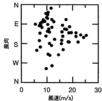
図-5 最大偏差発生時の風速と風向の関係
