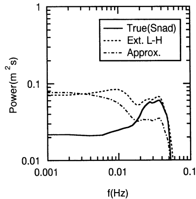
図-7 長周期拘束波のパワースペクトル ( S_{max}=75 )
