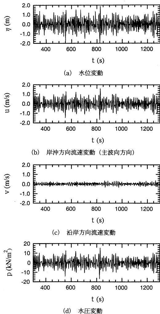
図一 シミュレートした基本波の波形の例 ( S_{max}=75 )
